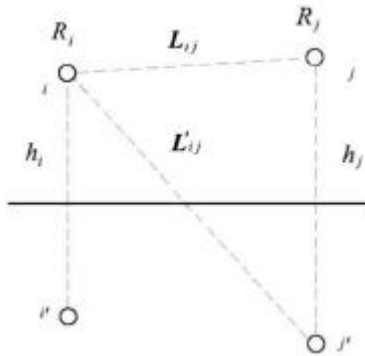
图 6-1 电位系数计算图
