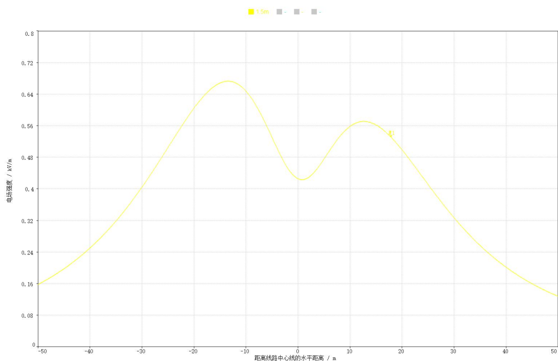
图 6-5 输电线路理论计算工频电场强度曲线图
