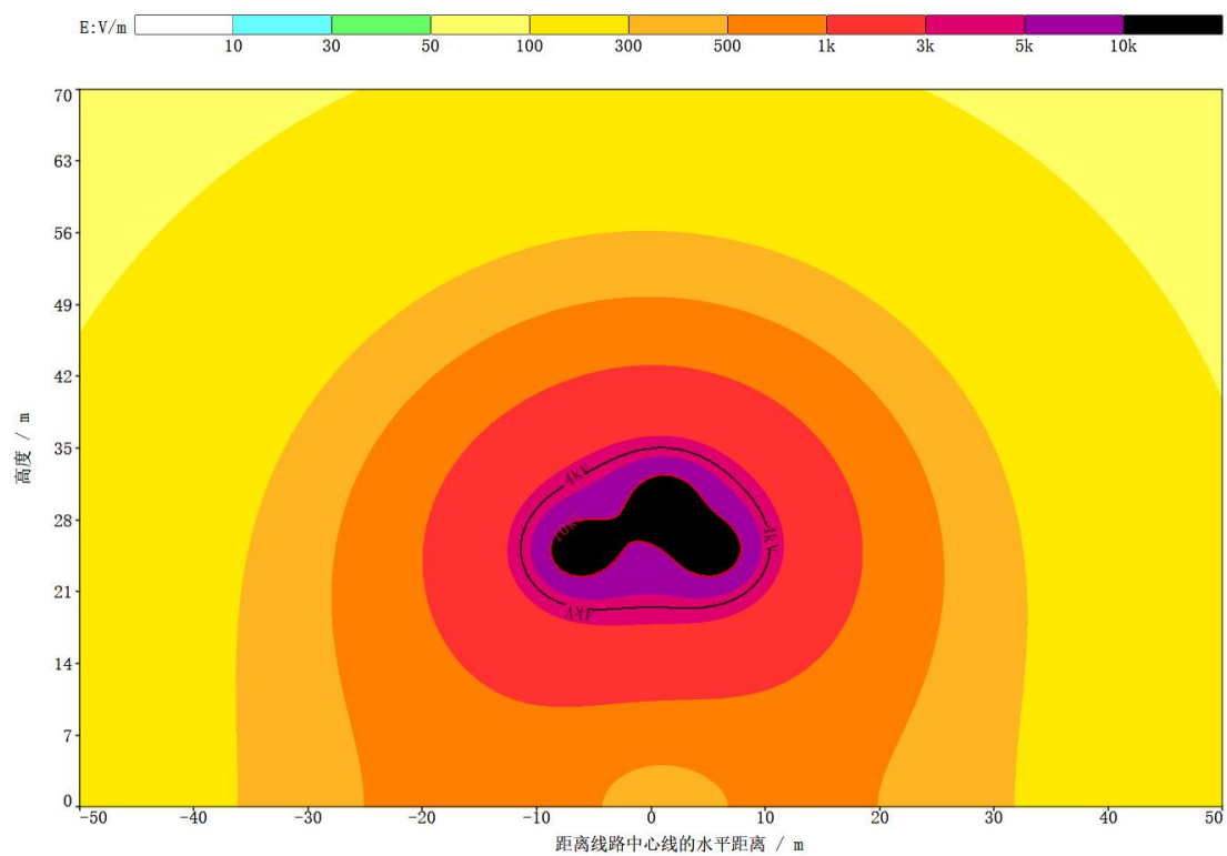
图 6-6 输电线路理论计算工频电场强度等值线图
