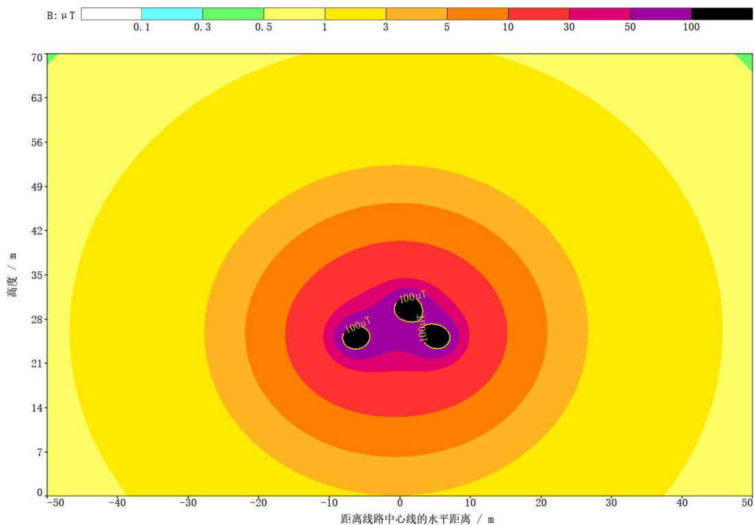
图 6-8 输电线路理论计算工频磁感应强度等值线图
