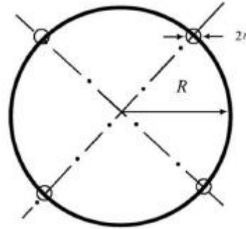
图 6-2 等效半径计算图
