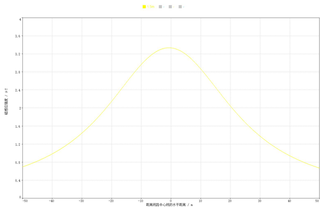
图 6-7 输电线路理论计算工频磁感应强度曲线图
