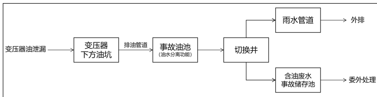
图 5-1 变压器事故排油处理流程图
